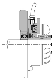
安裝于機台上的 NAB型制動器
