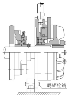
用轉矩栓銷來制動的 NAB型制動器
